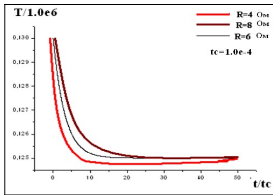
Рисунок 3 – Зависимость T от параметров установки
