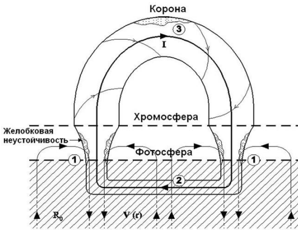
Рисунок 1 – Модель корональной арки с током
