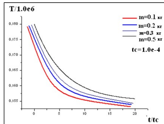
Рисунок 2 – Зависимость T от массы газа
